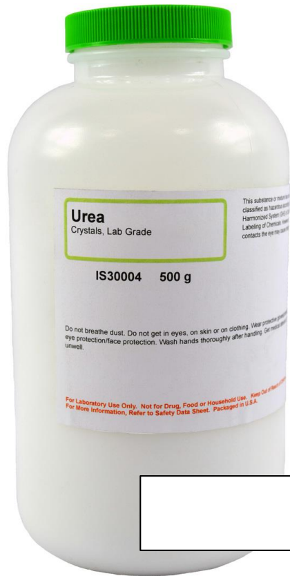
Urea
